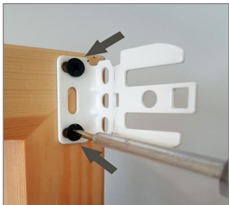
1. Metallträger an der Wand oder an der Decke anschrauben
